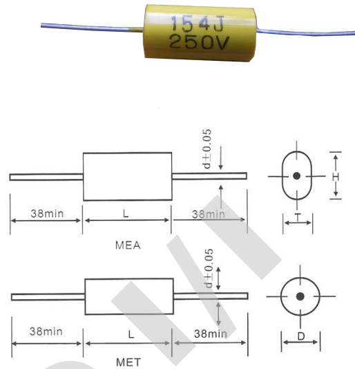
外形图 Outline Drawing
