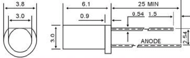
UNIT:mm
